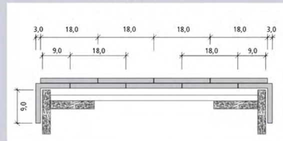
Secțiune longitudinală solzi STANDARD cu țiglă laterală
