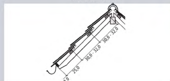
Așezare dublă solzi STANDARD
